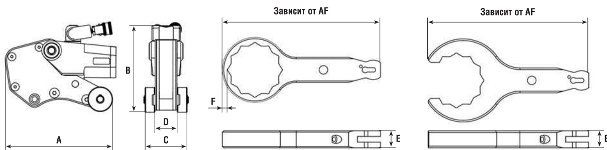
Привод с картрижем
